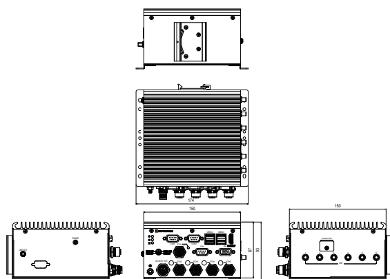
VBOX-3132P-M12X
