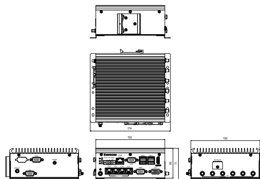
VBOX-3132P
