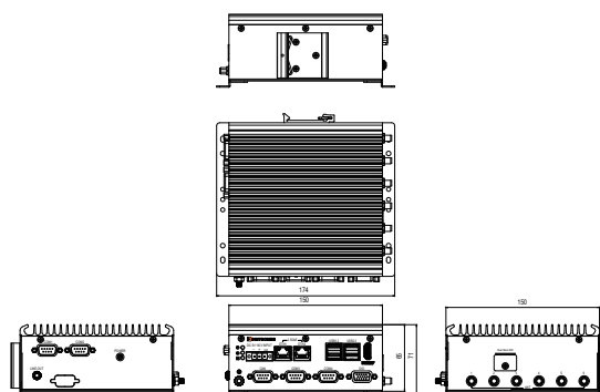
VBOX-3132-D25
