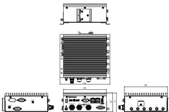
VBOX-3132-D25-M12X
